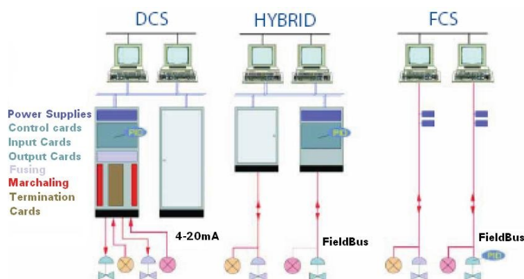
شکل ۱-۵ مقایسه ی ساختاری سیستم های کنترل DCS، FCS و Hybrid
