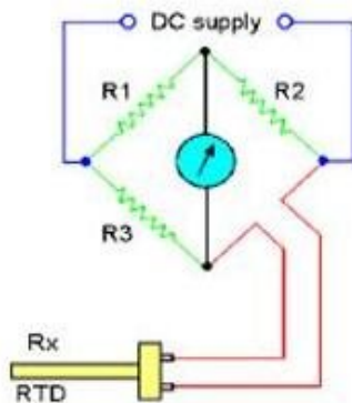
شکل ۳-۴ دما سنج RTD دوسیمه
